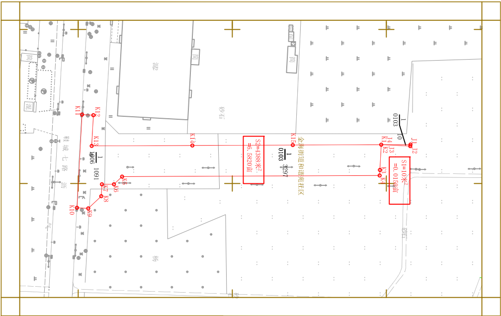
宿州市二〇二四年第一批次（增减挂钩）城市建设用地勘测定界简图（四）
